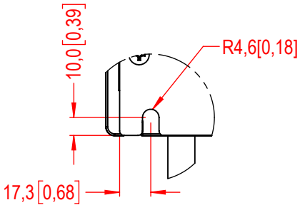
DETALHE / DETAIL B ESCALA / SCALE 1 : 3
