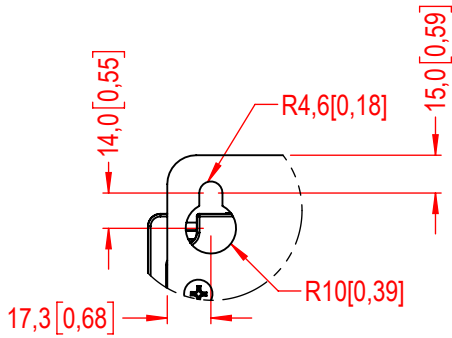
DETALHE / DETAIL A ESCALA / SCALE 1 : 3
